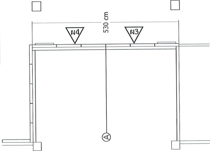
แบบขยายแบบครอบถ่ายภาพ
