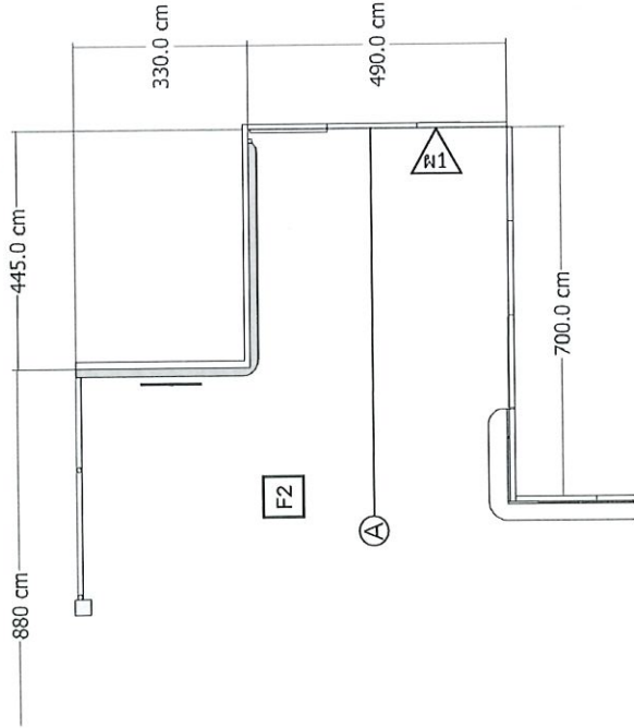
แบบขยายคลีนิกทันตกรรม top view
